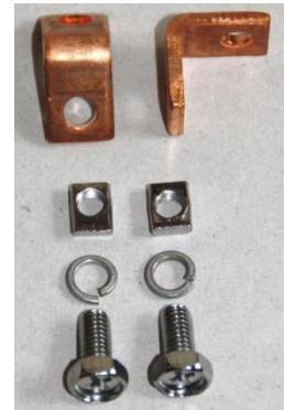
Batteriepol-Adaptersatz
